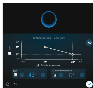
Optimální komfort a vysoká účinnost díky ekvitermní křivce, která automaticky upravuje požadovanou teplotu.
